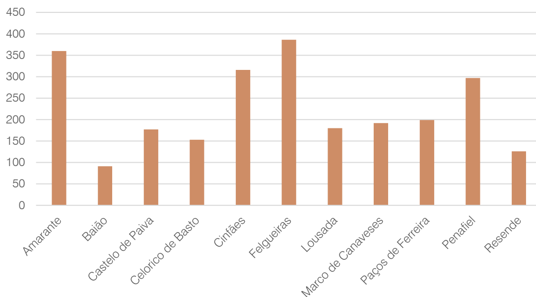
Figura 82. Número de ocorrências relacionadas com eventos de vento forte, nos municípios da CIM, no período 2013 – 2022
