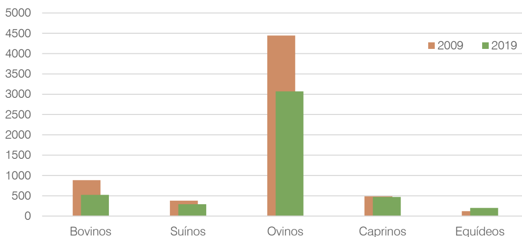
Figura 66. Efetivo Animal das Explorações Agrícolas em Marco de Canaveses (Nº de animais)
