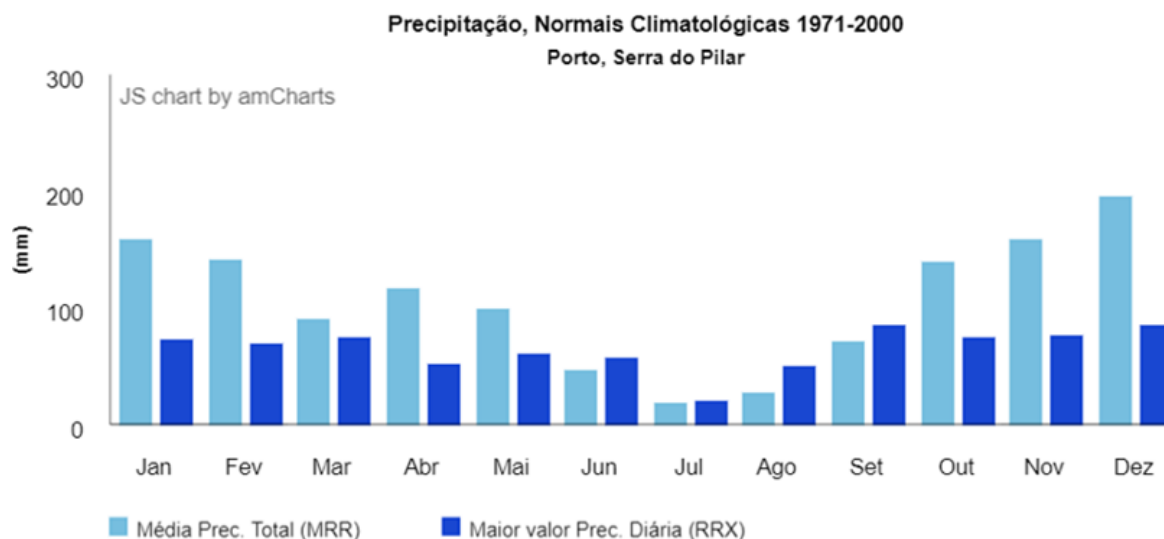
Figura 26. Precipitação segundo as normais climatológicas para o período 1971-2000 | Estação Meteorológica Porto/Serra do Pilar Fonte: IPMA
