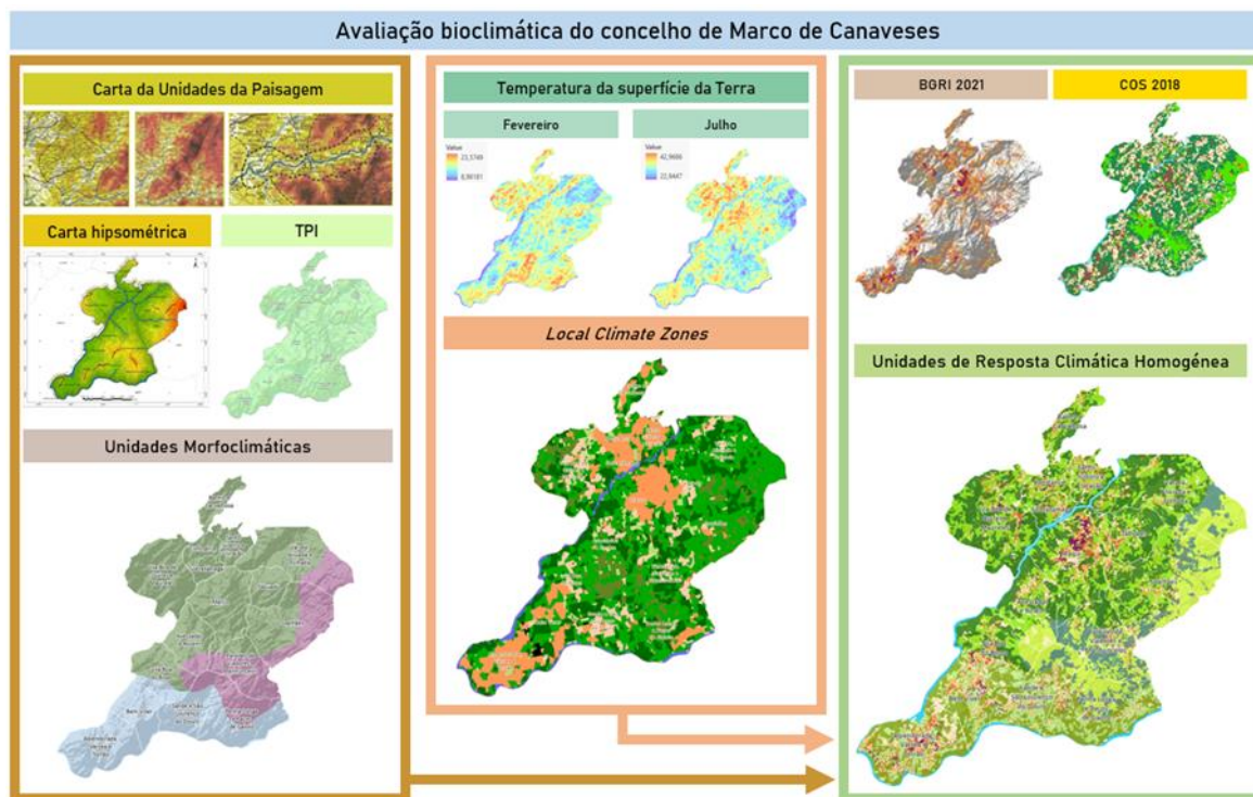
Figura 35. Metodologia para definição das UMC e URCH Fonte: SPI
