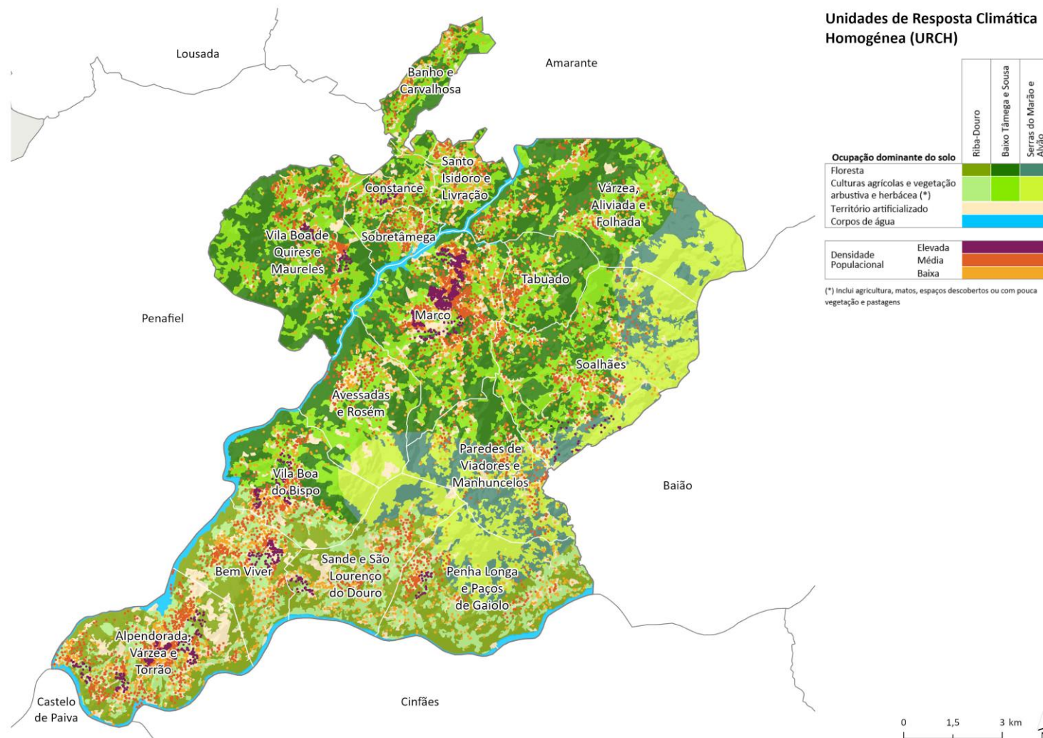
Figura 42. URCH do concelho de Marco de Canaveses
