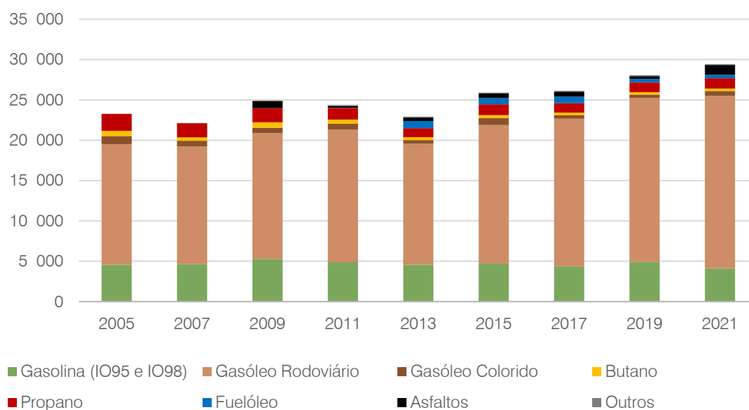
Figura 57. Evolução dos Consumos de Derivados de Petróleo, por vetor de consumo (ton) Fonte: DGEG
