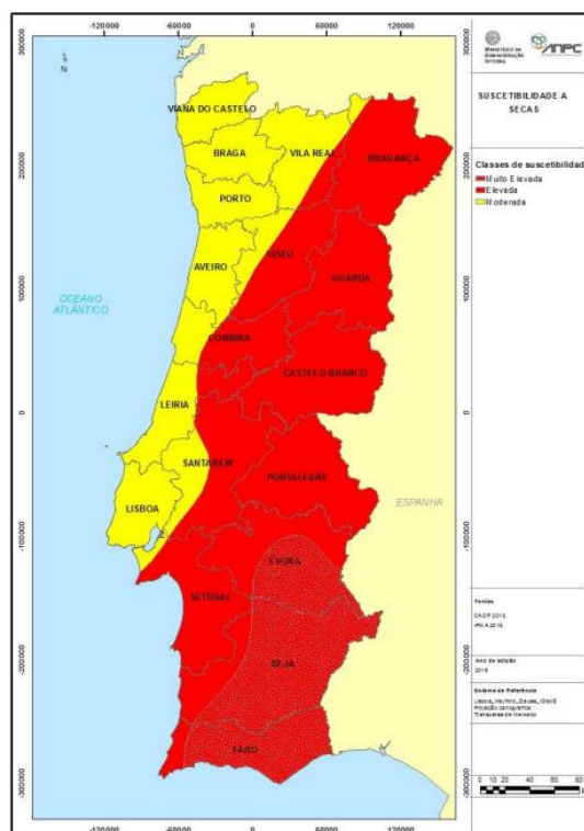
Figura 79. Carta de suscetibilidade a secas Fonte: IPMA apud PROCIV
