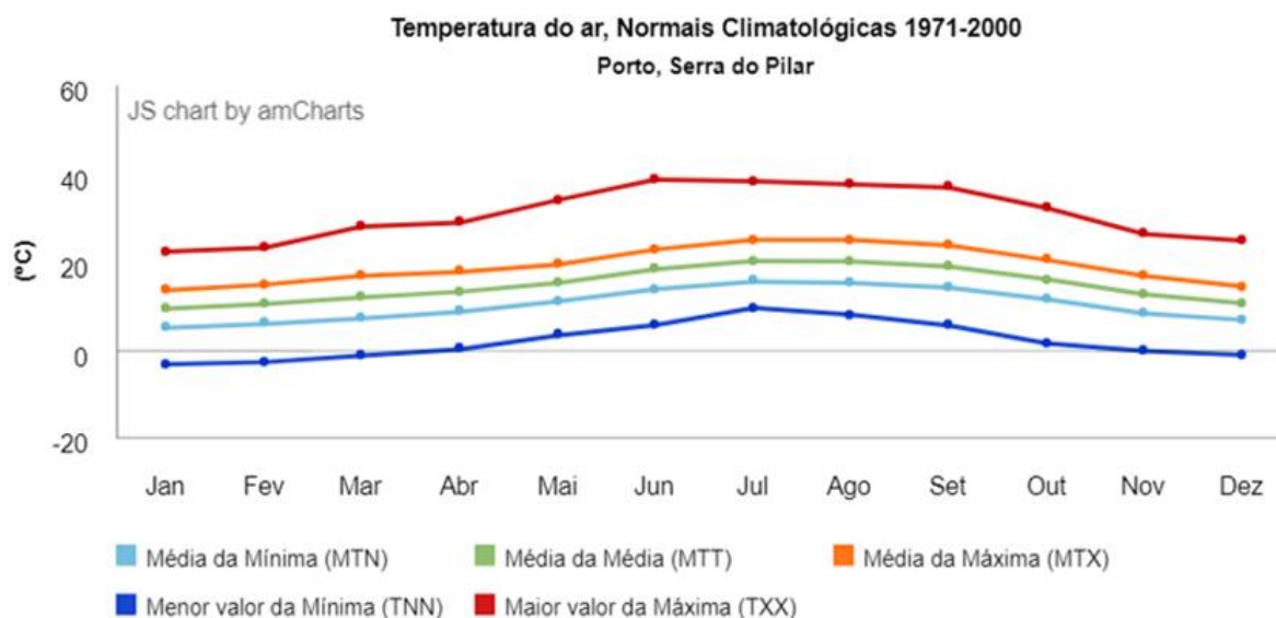
Figura 25. Temperatura do ar segundo as normais climatológicas para o período 1971-2000 | Estação Meteorológica do Porto/Serra do Pilar Fonte: IPMA
