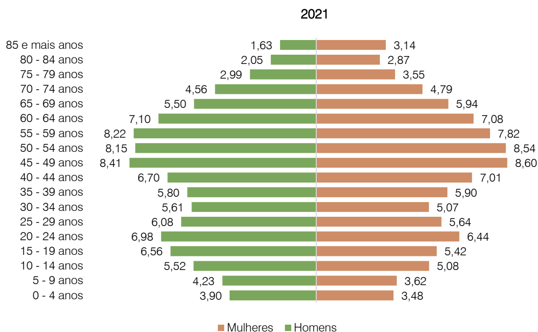
Figura 19. Pirâmide etária do concelho em 2021
