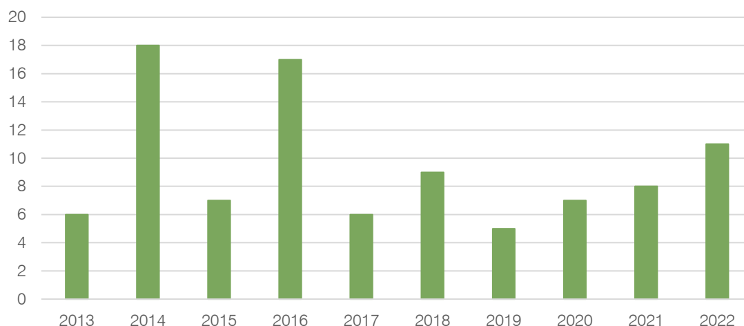
Figura 76. Distribuição anual do número de dias com precipitação excessiva
