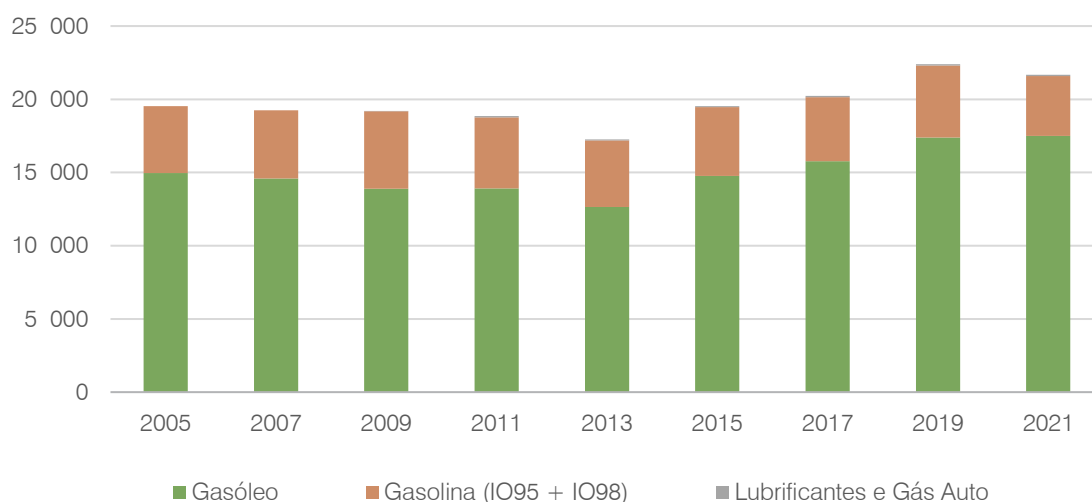
Figura 58. Consumo de Derivados de Petróleo para Transportes (ton.) Fonte: DGEG
