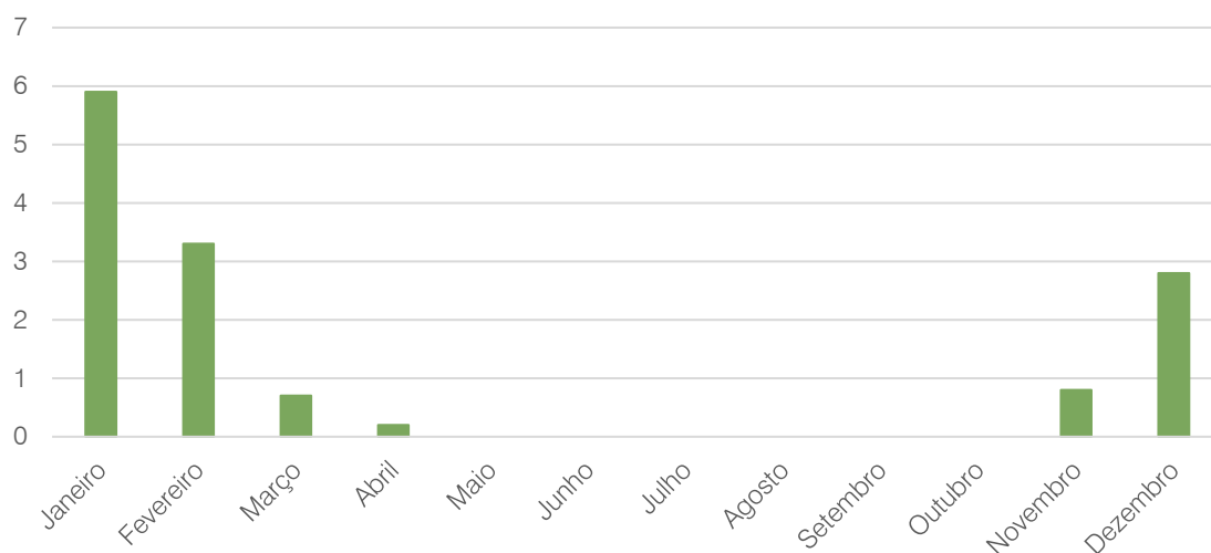
Figura 84. Número médio mensal de dias com temperatura abaixo de 0°C (2013-2022) Fonte: IPMA
