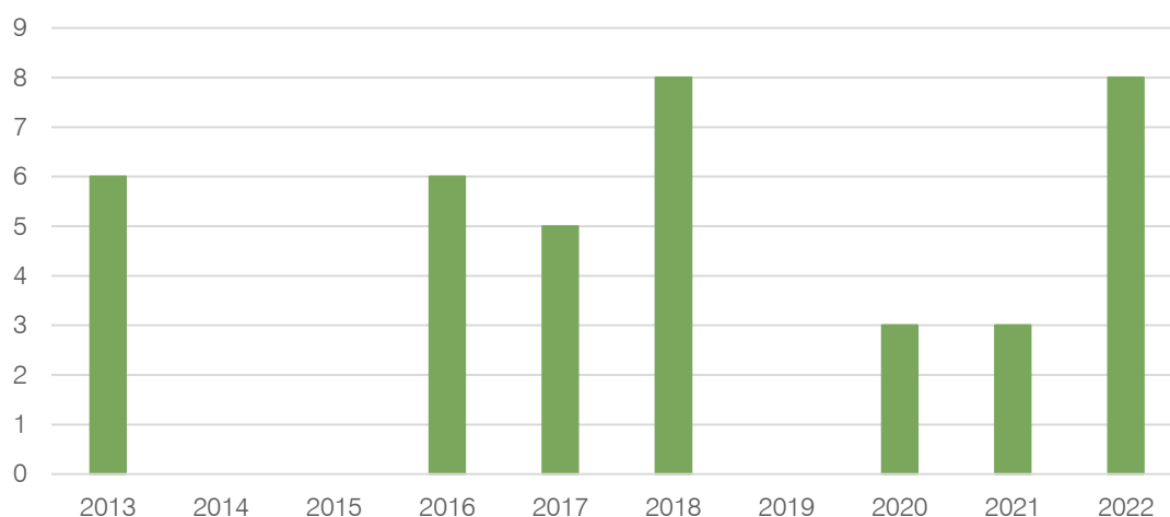
Figura 74. Número de dias com temperaturas >35° em cada ano Fonte: IPMA
