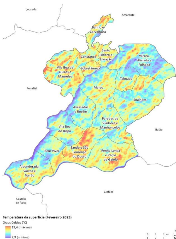
Figura 41. Temperatura da superfície do concelho de Marco de Canaveses em fevereiro de 2023 Fonte: Landsat 8-9 OLI/TIRS C2 L1
