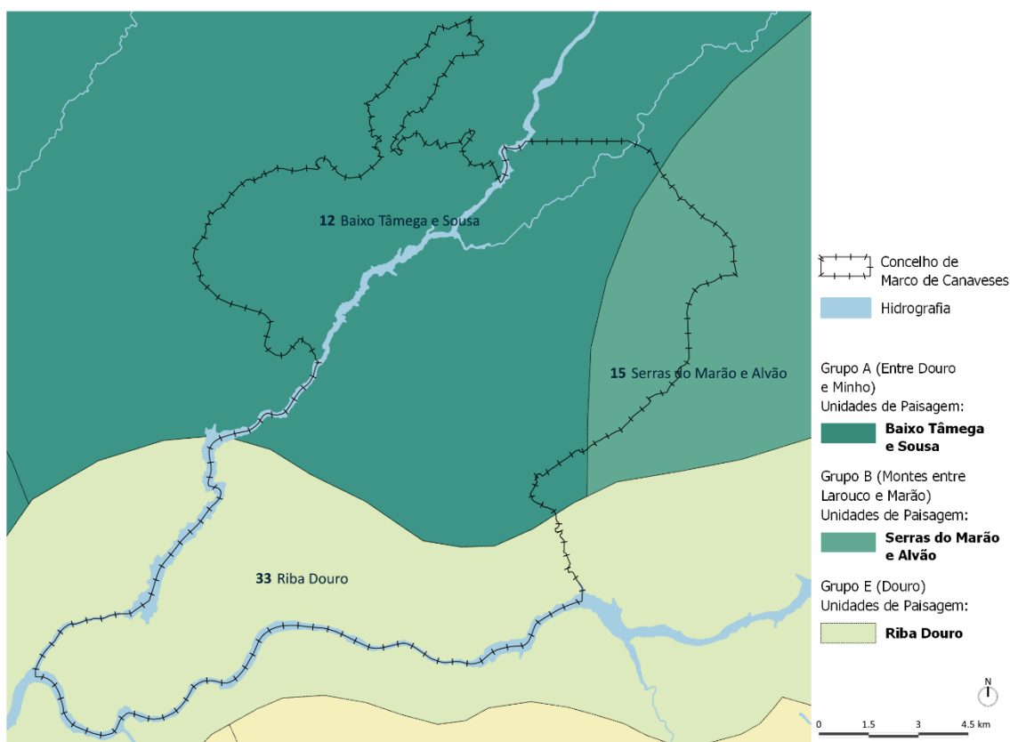
Figura 21. Unidades de paisagem do município de Marco de Canaveses Fonte: Direção Geral do Território (2004)
