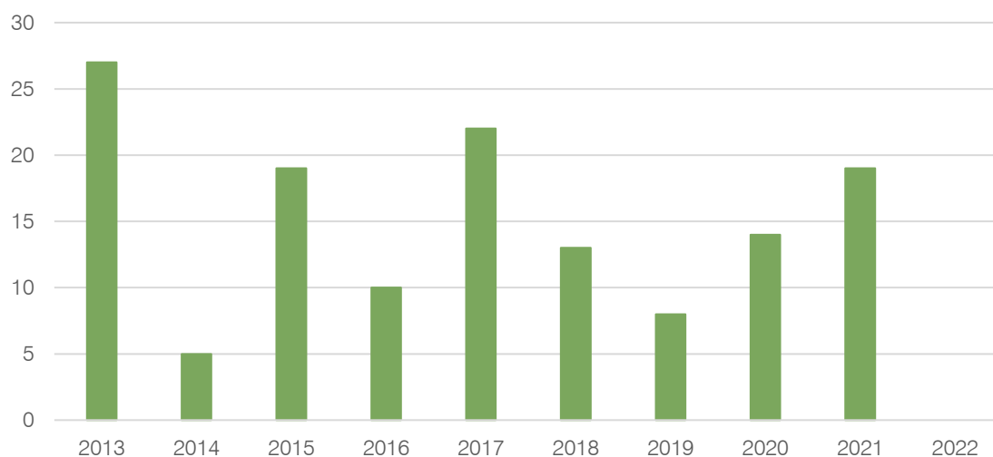
Figura 85. Número de dias com temperaturas negativas em cada ano, no período em análise Fonte: IPMA
