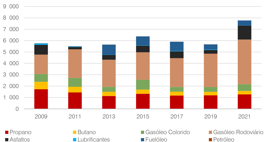
Figura 59. Evolução do Consumo de Derivados de Petróleo (toneladas)
