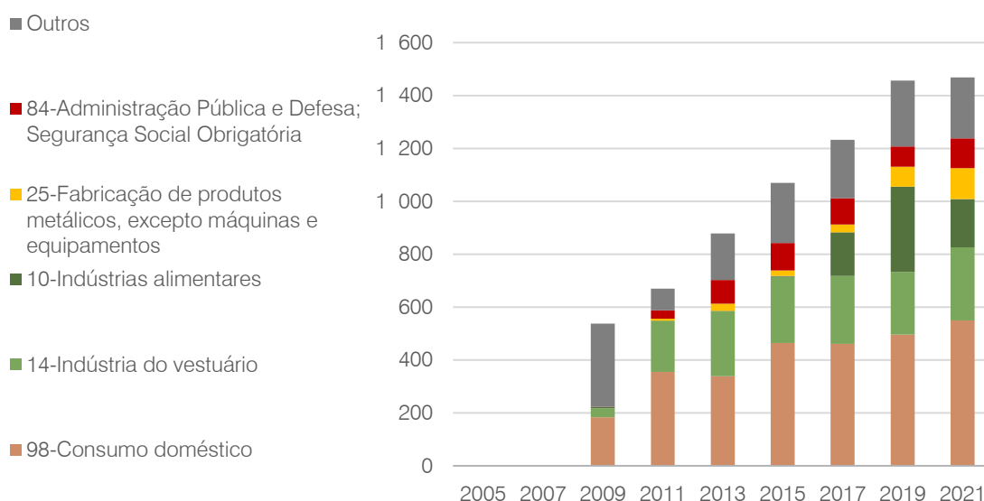
Figura 61. Evolução do Consumo de Gás Natural (10³Nm³) Fonte: DGEG
