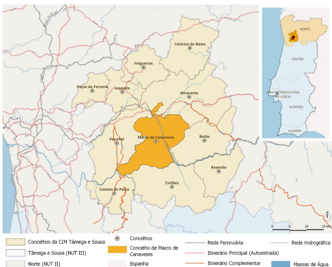
Figura 15. Enquadramento do município de Marco de Canaveses na CIM-TS
