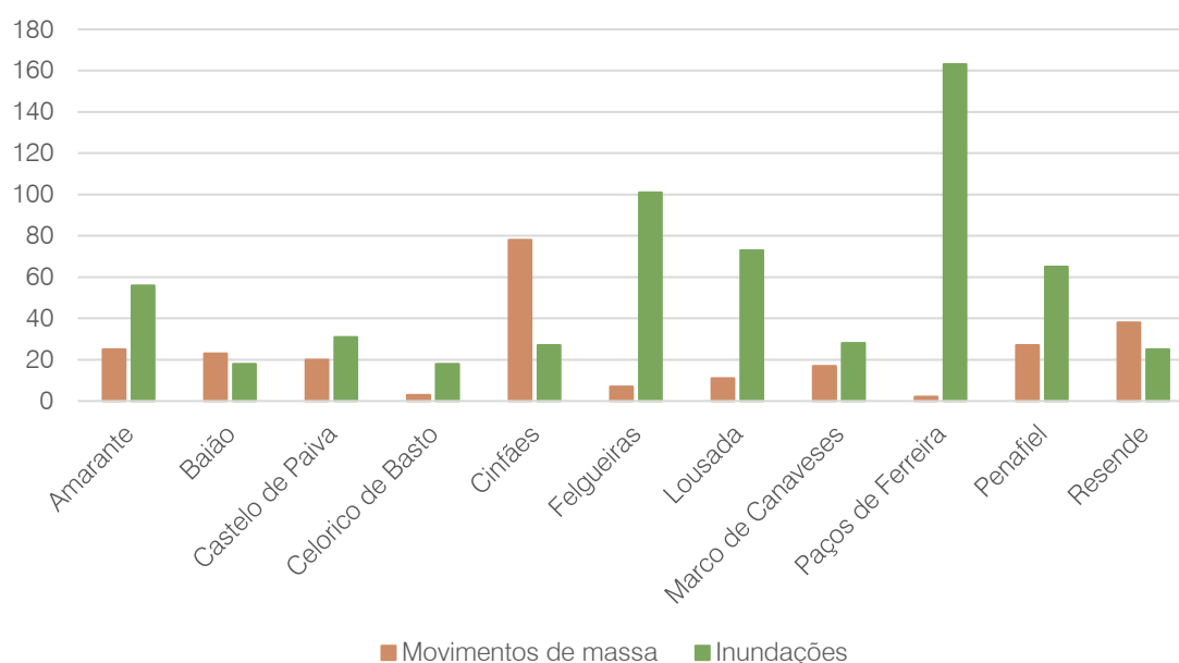
Figura 78. Número de ocorrências relacionadas com eventos de precipitação excessiva, nos municípios da CIM, no período 2013 – 2022
