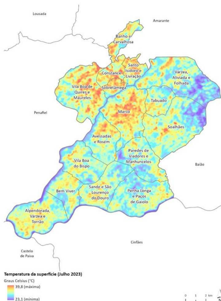
Figura 40. Temperatura da superfície do concelho de Marco de Canaveses em julho de 2023 Fonte: Landsat 8-9 OLI/TIRS C2 L1
