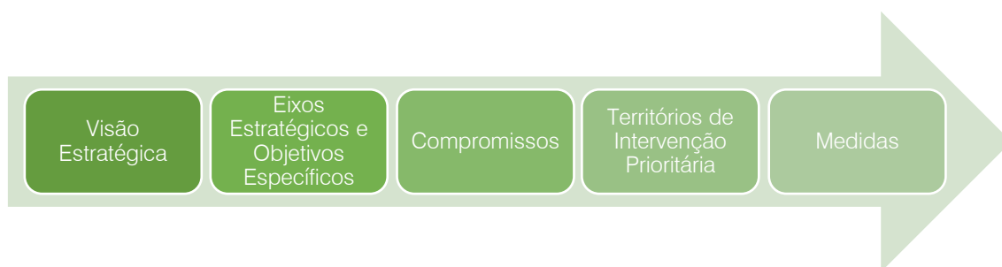
Figura 86. Níveis de definição estratégica
