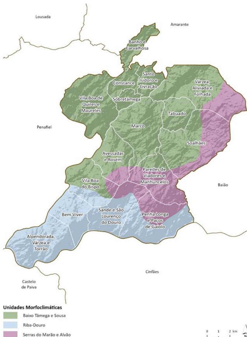
Figura 37. Unidades morfoclimáticas do concelho de Marco de Canaveses Fonte: SPI
