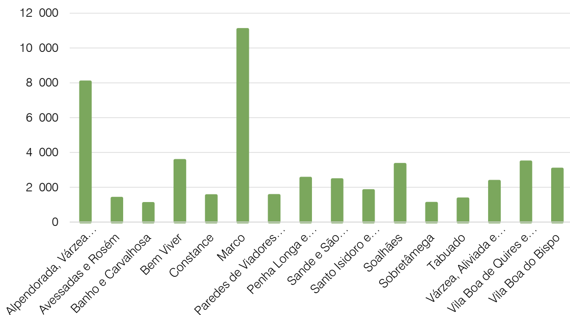
Figura 17. Distribuição da população residente pelas freguesias de Marco de Canaveses em 2021 Fonte: INE
