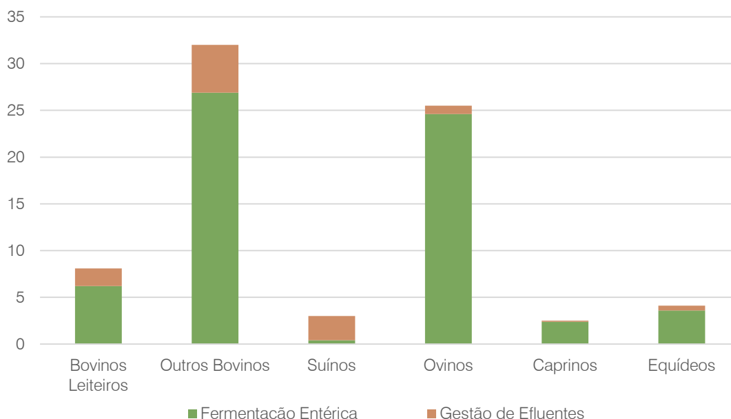
Figura 67. Emissões de CH 4 por tipo de gado e processo de libertação de GEE (ton. CH 4 ) (2019)
