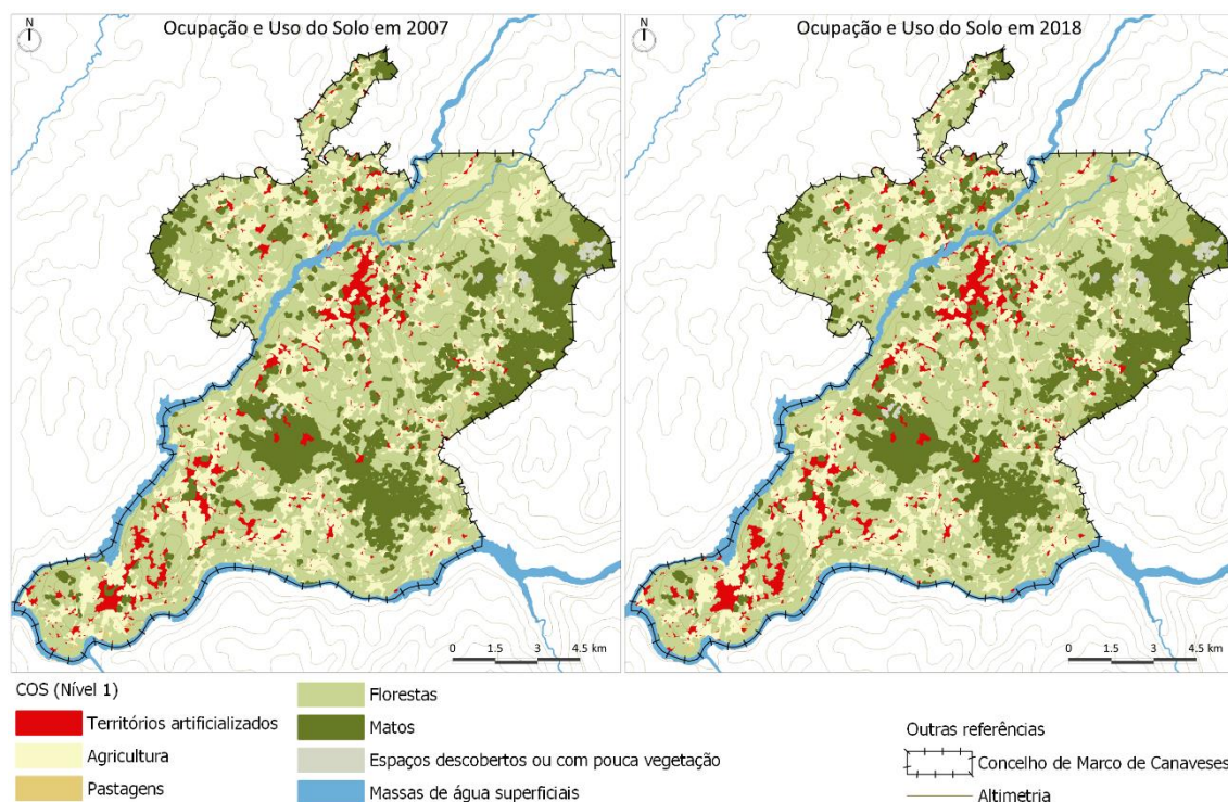
Figura 68. Evolução do uso do solo no concelho do Marco de Canaveses - COS 2007 e 2018 (Nível I) Fonte: Direção Geral do Território (2023)
