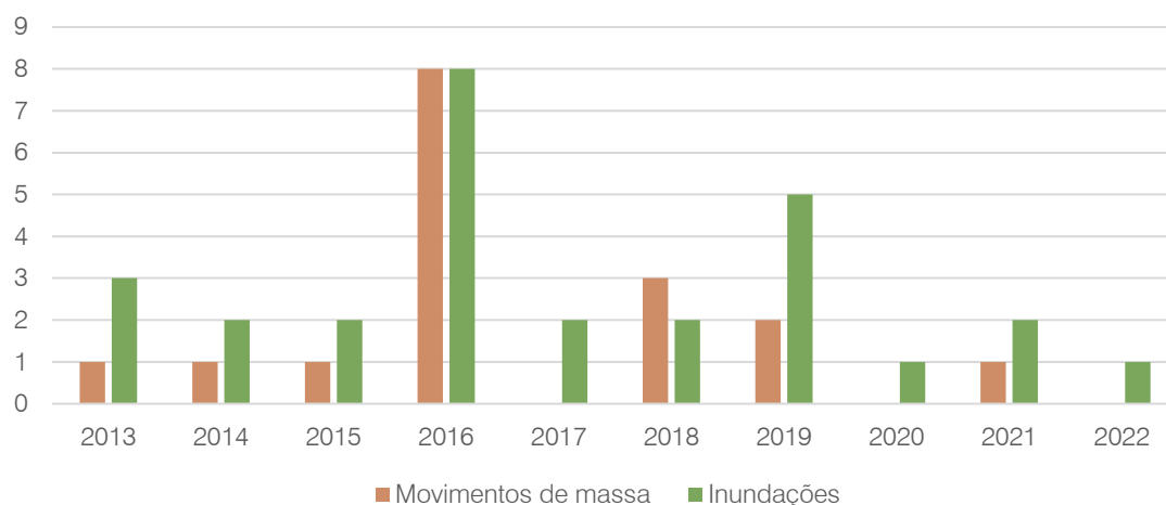
Figura 77. Número de ocorrências relacionadas com eventos de precipitação excessiva em Marco de Canaveses (2013-2022)
