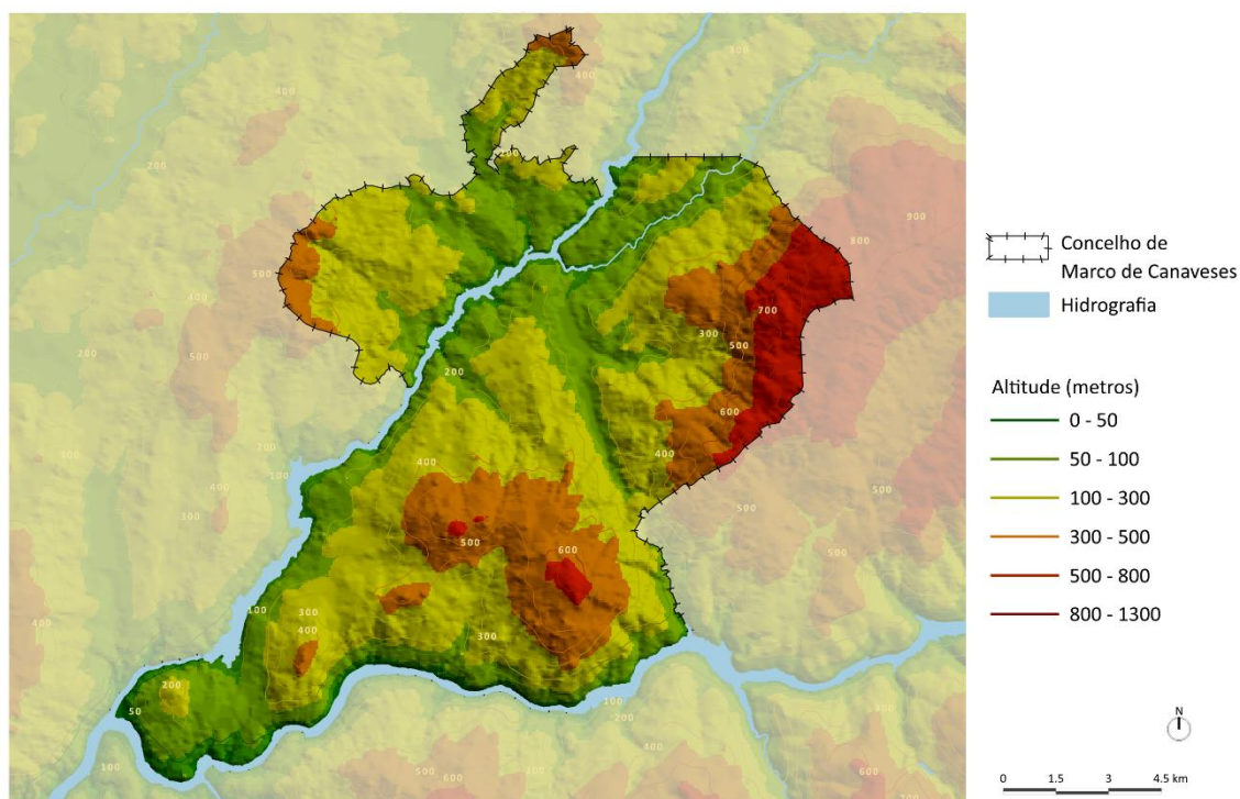
Figura 20. Mapa hipsométrico do município de Marco de Canaveses
