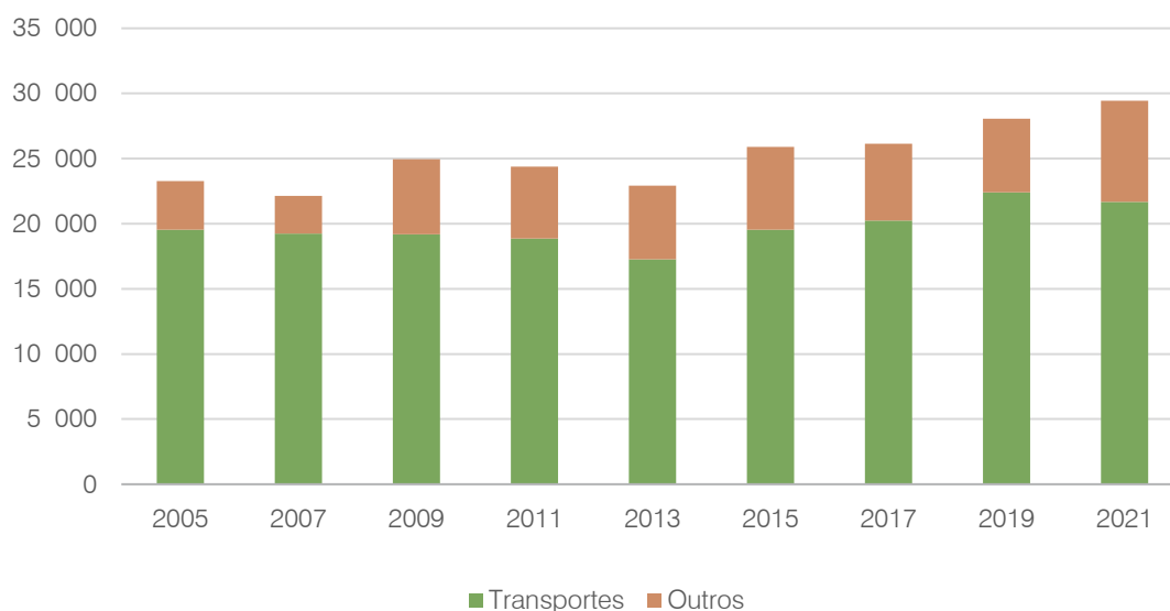
Figura 55. Evolução dos Consumos de Derivados de Petróleo, por atividade (ton) 29 Fonte: DGEG
