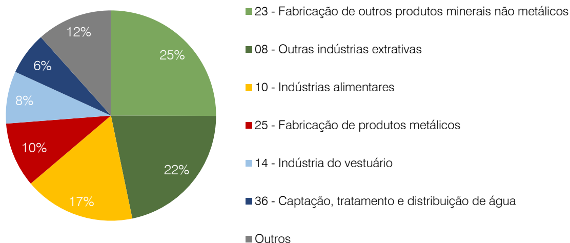
Figura 52. Análise dos Consumos Industriais de Energia Elétrica (2021) Fonte: DGEG
