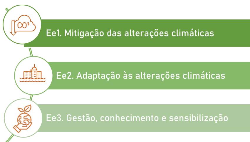
Figura 87. Eixos Estratégicos para a Ação Climática
