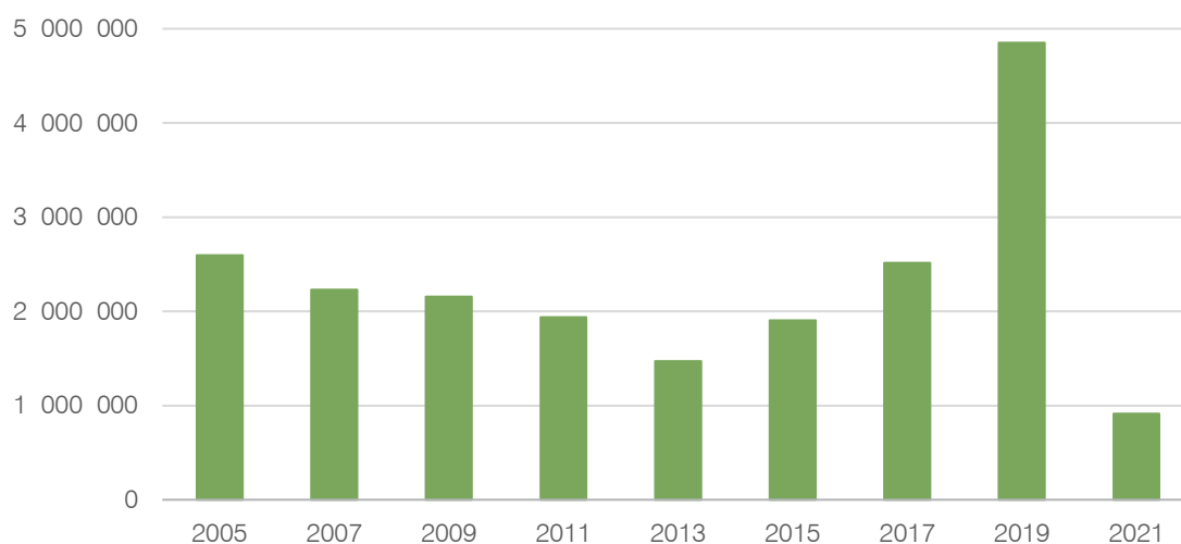
Figura 54. Consumo Agrícola de Eletricidade (kWh)
