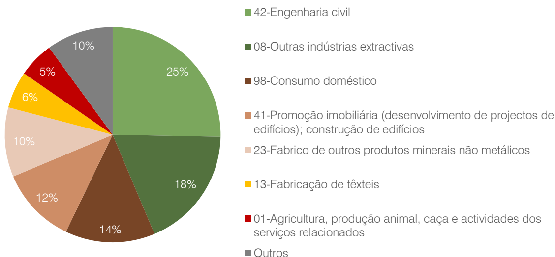
Figura 60. Distribuição do consumo de Derivados de Petróleo por atividade económica, exceto transportes (2021)
