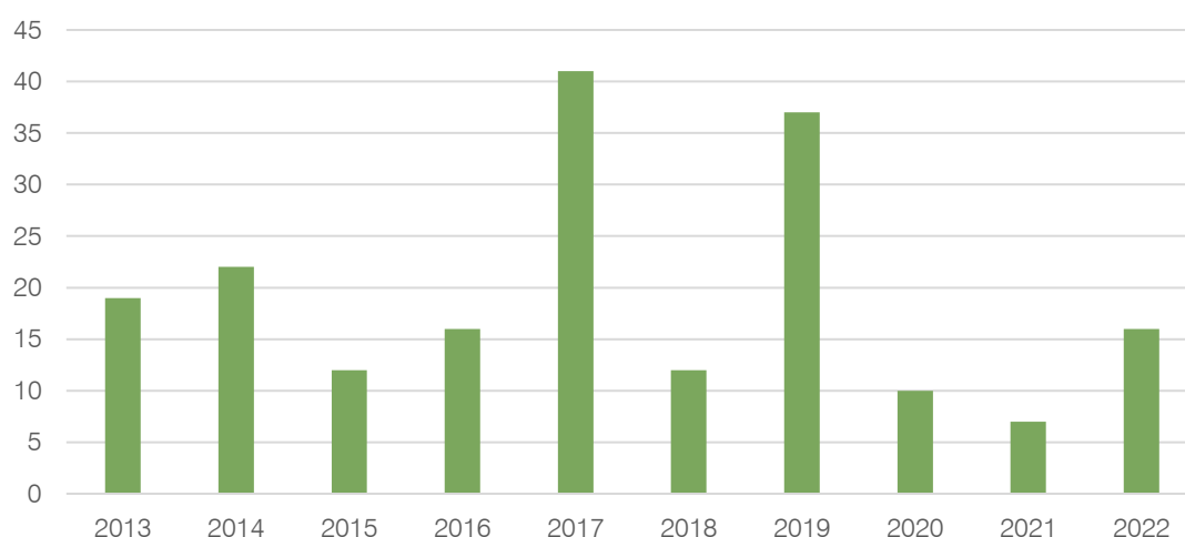
Figura 81. Número de ocorrências relacionadas com eventos de vento forte em Marco de Canaveses (2013-2022)
