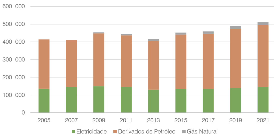
Figura 43. Evolução dos Consumos Energéticos no Marco de Canaveses entre 2005 e 2021 (MWh) Fonte: DGE
