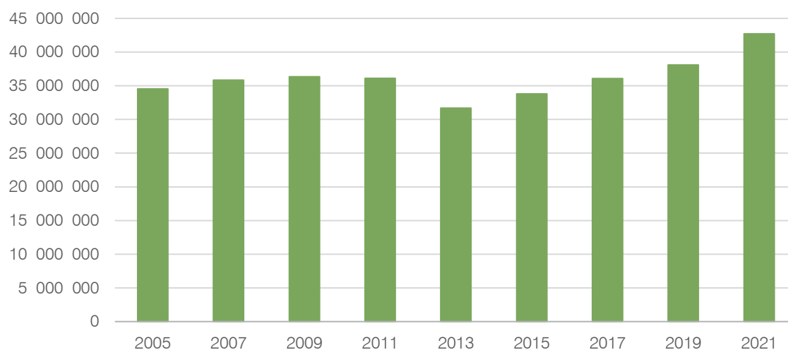
Figura 51. Consumo industrial de eletricidade (kWh)
