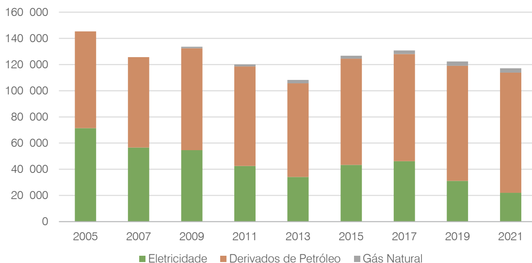
Figura 62. Evolução Temporal das Emissões de GEE (toneladas CO 2eq )
