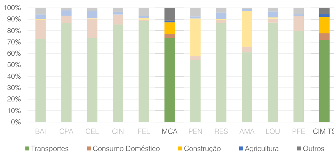
Figura 56. Comparação da Distribuição dos Consumos de Derivados de Petróleo por Atividade Económica, nos Vários Concelhos do Tâmega e Sousa (2021) Fonte: DGEG
