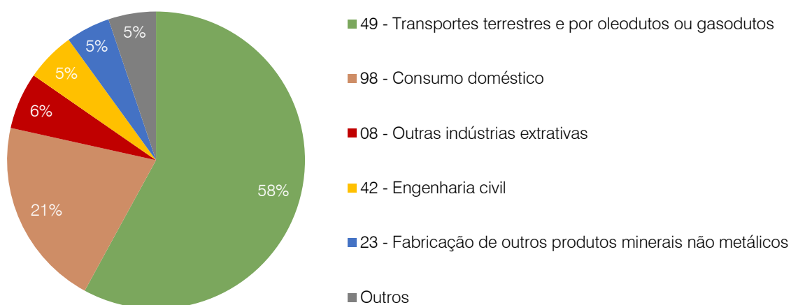
Figura 63. Distribuição das Emissões de GEE por atividade económica (2021)
