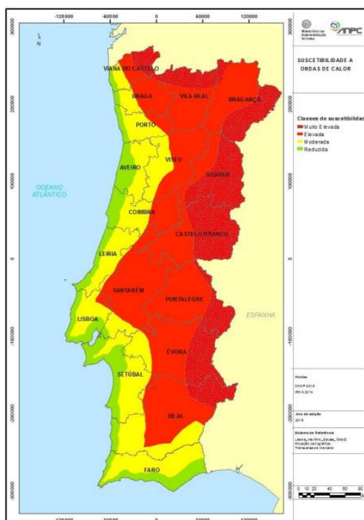
Figura 71. Carta de suscetibilidade a ondas de calor Fonte: Adaptado de IPMA apud PROCIV
