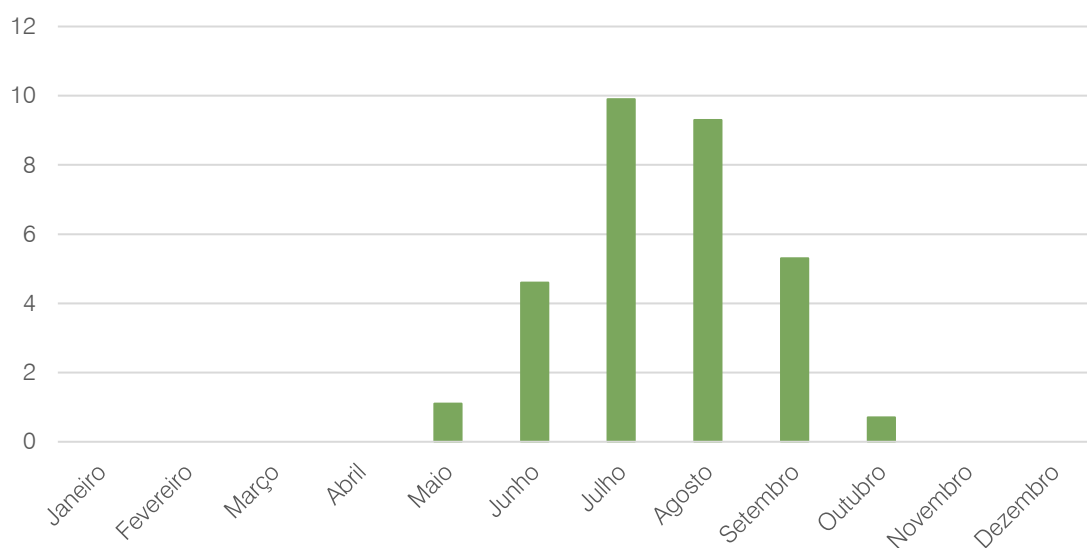
Figura 72. Número médio mensal de dias com temperatura >30°C, (2013-2022) Fonte: IPMA
