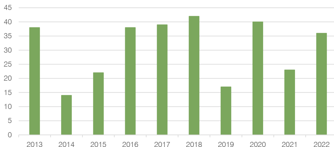
Figura 73. Número de dias com temperaturas >30° em cada ano Fonte: IPMA
