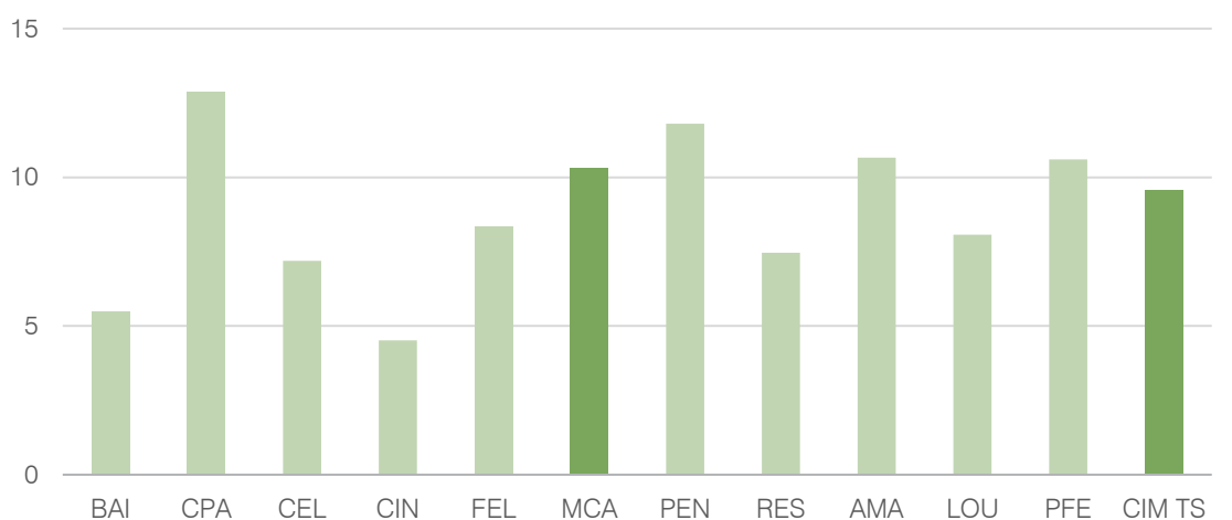
Figura 45. Consumos per Capita de Energia, na região do Tâmega e Sousa, em 2021 (MWh / hab.) Fonte: DGEG / INE
