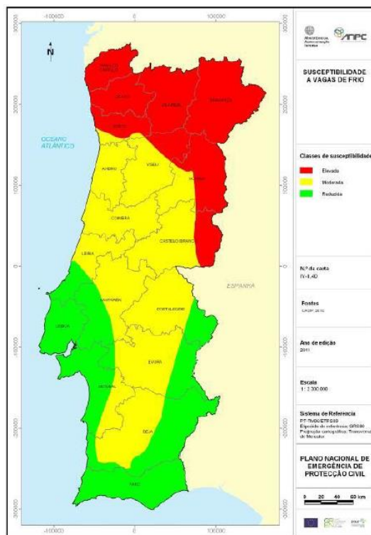
Figura 83. Carta de suscetibilidade a ondas de frio Fonte: ANPC apud PROCIV
