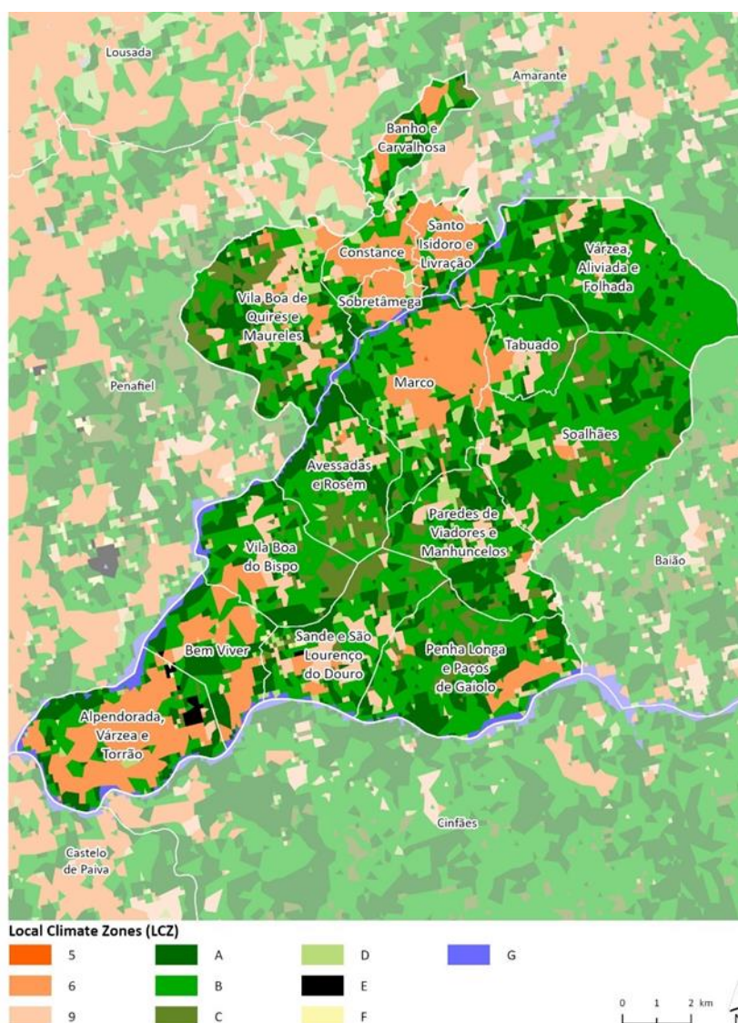
Figura 39. Local Climate Zones (LCZ) do concelho de Marco de Canaveses Fonte: SPI, com base em WUDAPT, 2023
