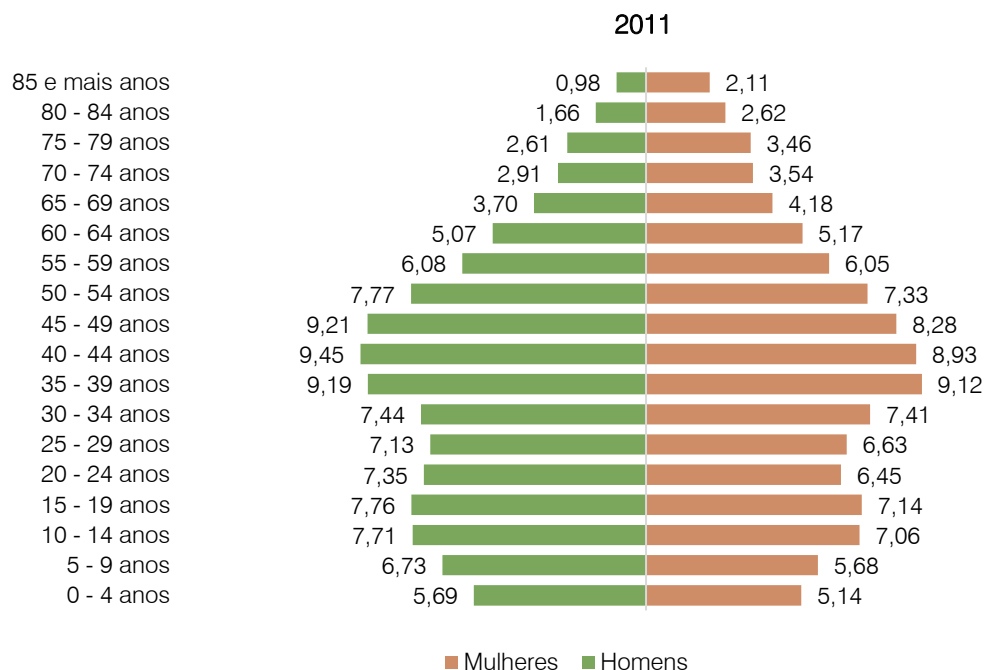
Figura 18. Pirâmide etária do concelho em 2011 Fonte: INE
