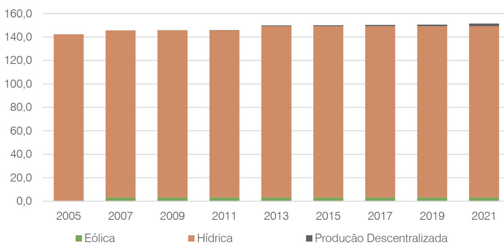
Figura 64. Evolução da Potência Instalada em Fontes de Energia Renovável (MW) Fonte: DGEG
