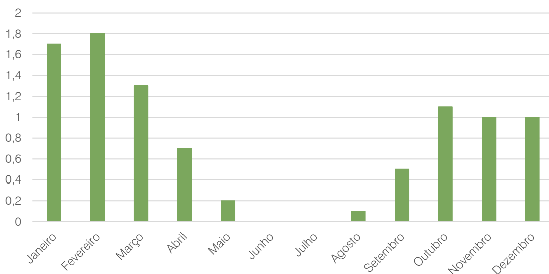
Figura 75. Distribuição do número médio de dias com precipitação excessiva, por mês (2013-2022) Fonte: IPMA
